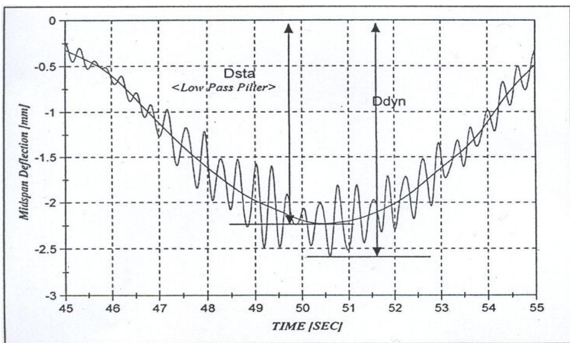
【그림 4.1-10】 처짐이력곡선
